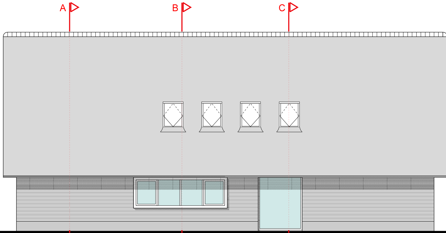
rechtergevel
