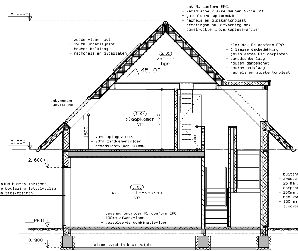
doorsnede A - A
