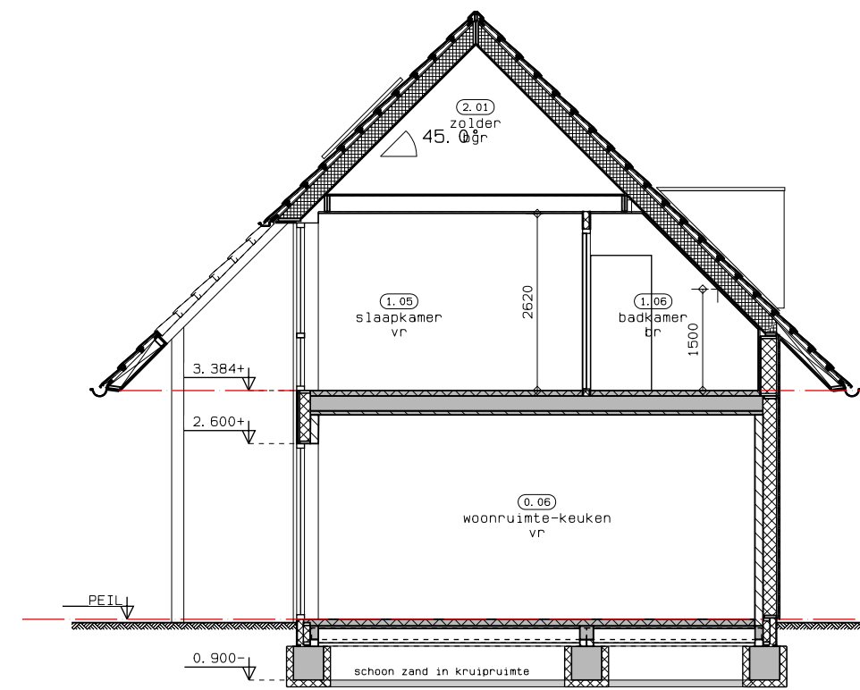
doorsnede B - B
